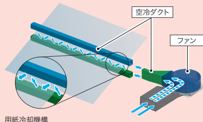
用紙冷却機構
